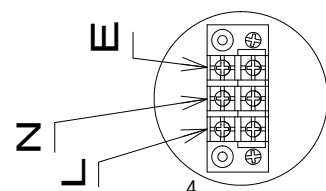
詳細図A 電源入力
