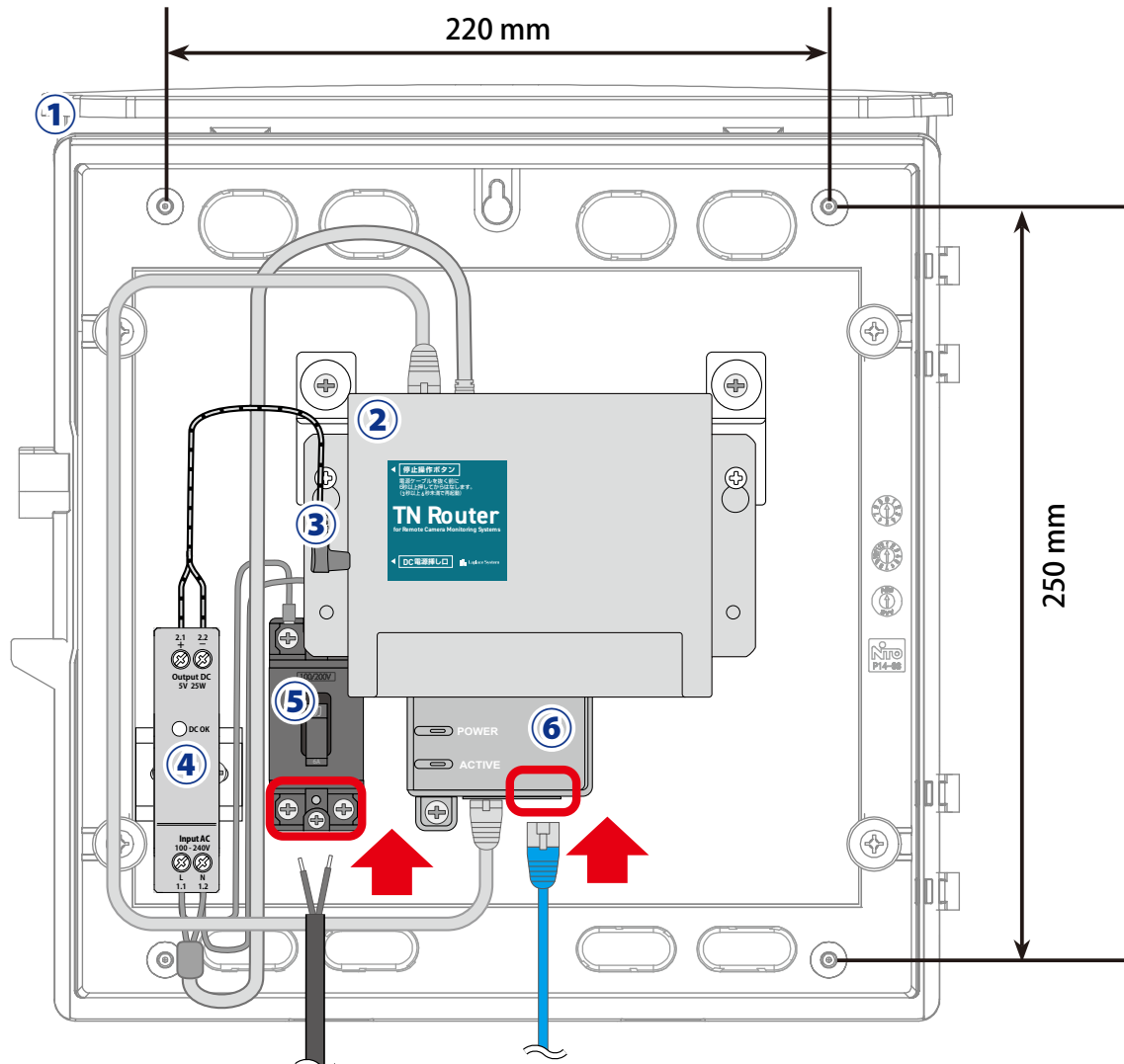
電源用ケーブル (AC100V/200V) Web カメラ接続用 LAN ケーブル
