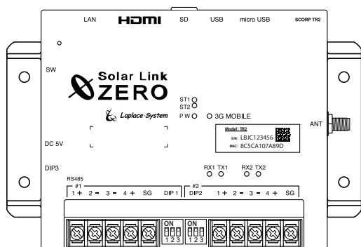
① Solar Link ZERO 本体 (以下、ZERO 本体)
