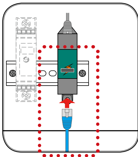
パワーコンディショナなどからの LAN ケーブル
