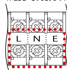
電源ケーブル接続箇所
