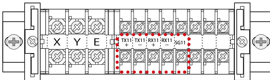
パワーコンディショナからの 信号線接続箇所
