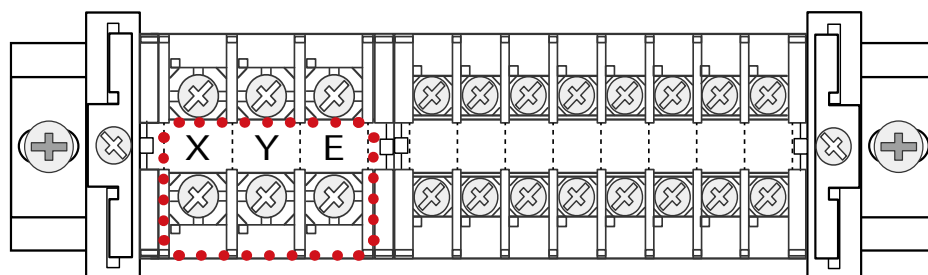
AC 電源接続箇所
